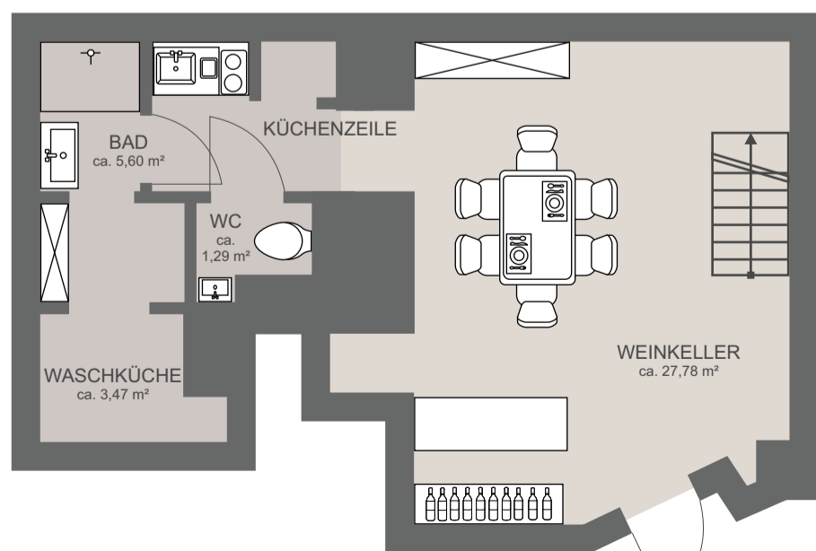
KELLERGESCHOSS
