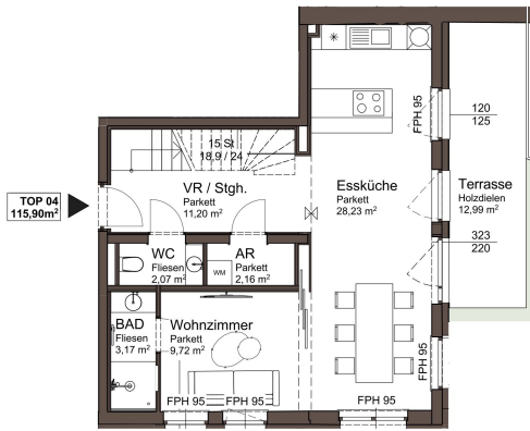
ERDGESCHOSS
