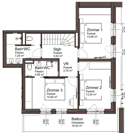
1. OBERGESCHOSS
