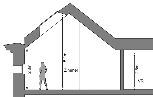
Schnitt B
