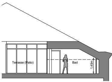
Schnitt B
