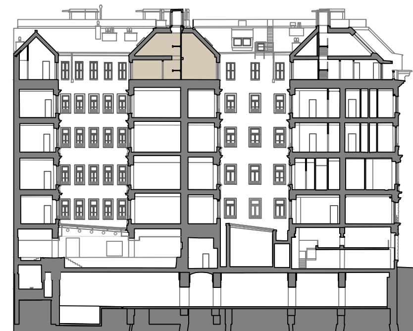
SNITT E-E
