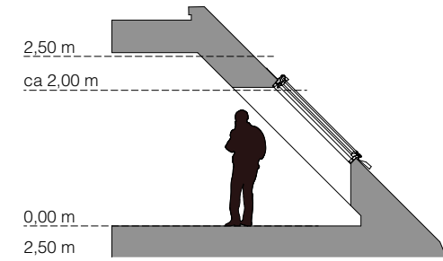
Systemschnitt c-c
