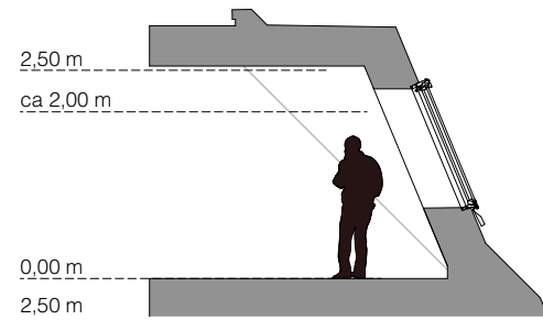
Systemschnitt a-a
